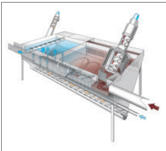
Principio de funcionamiento Ro5 HD
